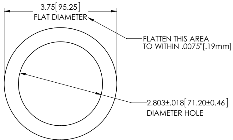
H.V. TANK HOLE DIMENSIONS
